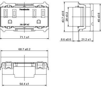
埋入式5.5mm 2 絞線用瞬瞬附接地極插座
