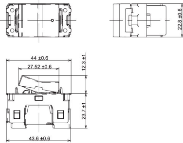
埋入式瞬瞬附接地極雙插座
