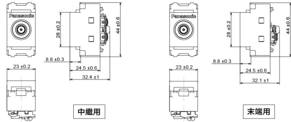
埋入式電視機插座(中繼&端末用)
