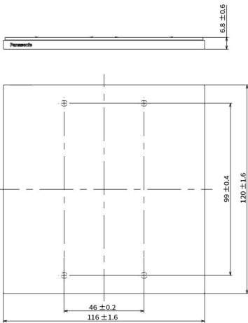
封口蓋板 (2連用)(附安裝框)
