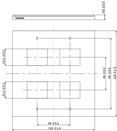
蓋板 (4個用)(附安裝框)
