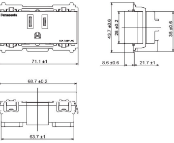
埋入式瞬瞬15A・20A附接地極插座
