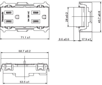
埋入式5.5mm 2 絞線用瞬瞬附接地極雙插座
