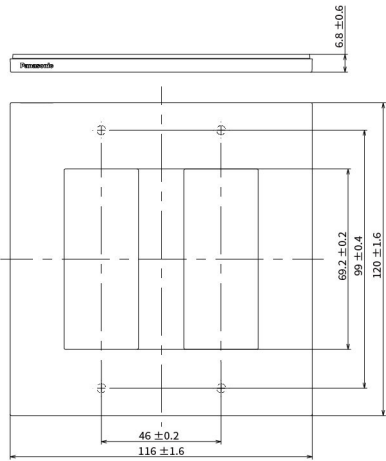
蓋板 (6個用)(附安裝框)
